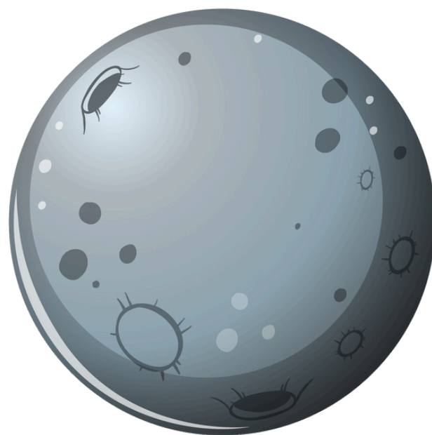
Moon
